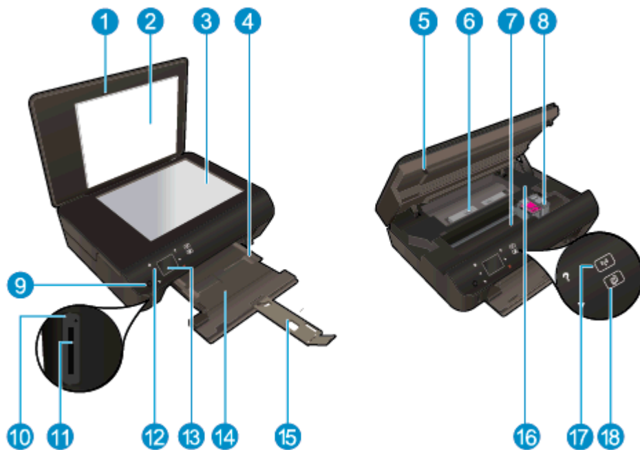
图 2-1 HP ENVY 5530 e-All-in-One Series 的前视图和上视图
