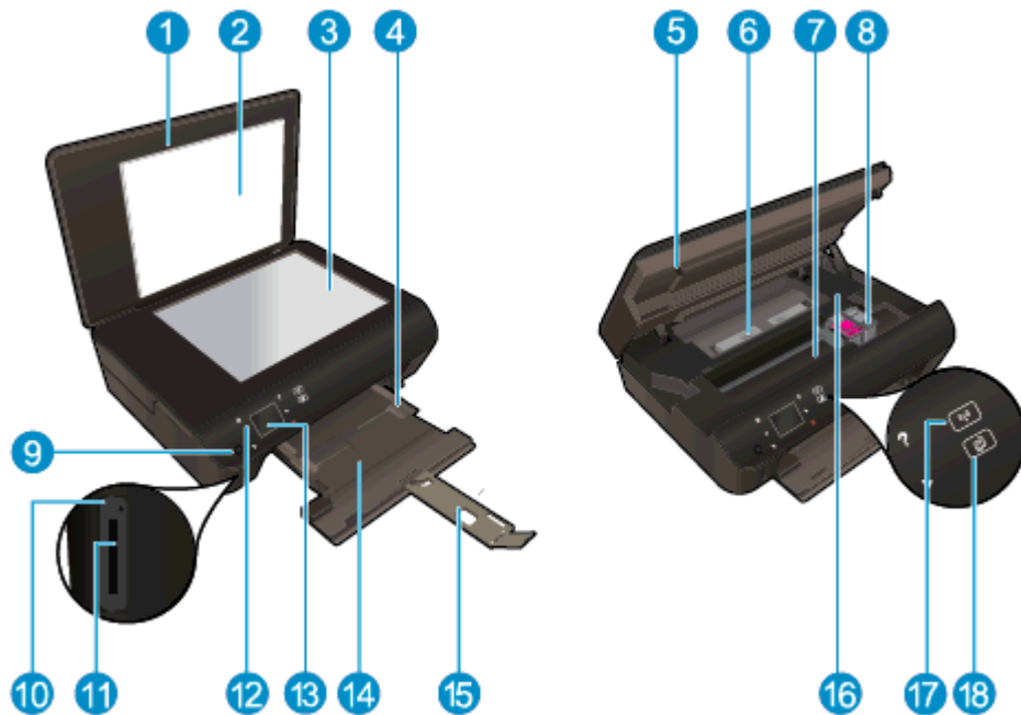
Rysunek 2-1 Widok urządzenia HP Deskjet Ink Advantage 4510 e-All-in-One Printer z przodu i z góry
