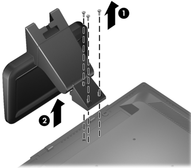
Figura 2-7 Extracción de la base del pedestal
