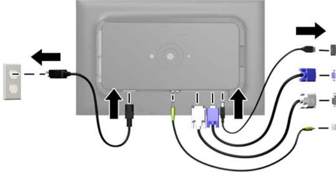
Şekil 3-4 Kabloları Bağlama
