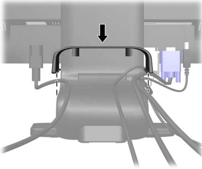
Şekil 3-5 Kablo Yönetim Klipsini Takma
