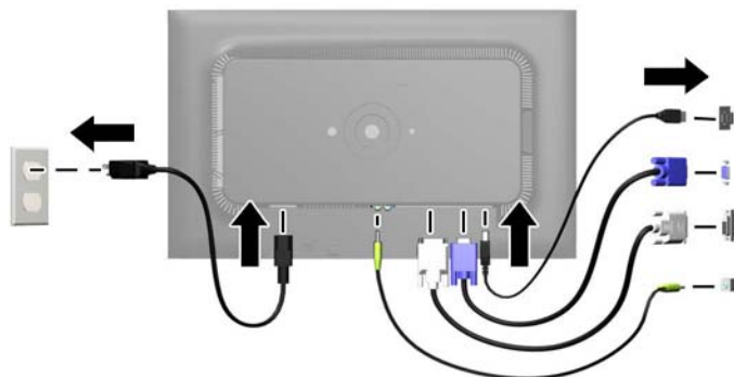
Obrázek 3-4 Připojení kabelů
