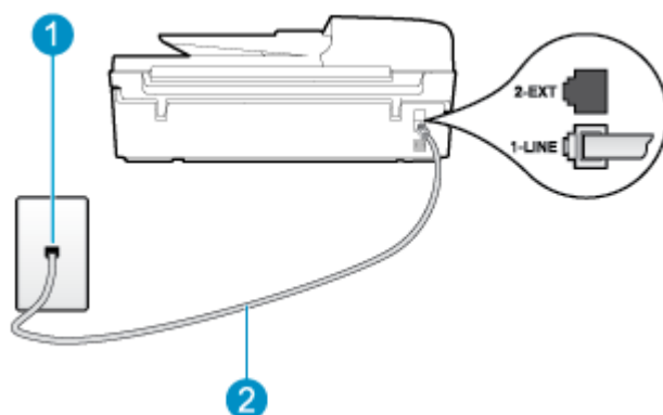
איור ב-1 מראה המדפסת מאחור
