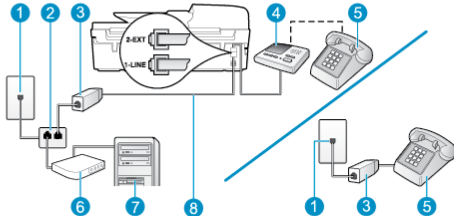
איור ב-15 מראה המדפסת מאחור
