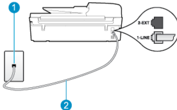
איור ב-5 מראה המדפסת מאחור
