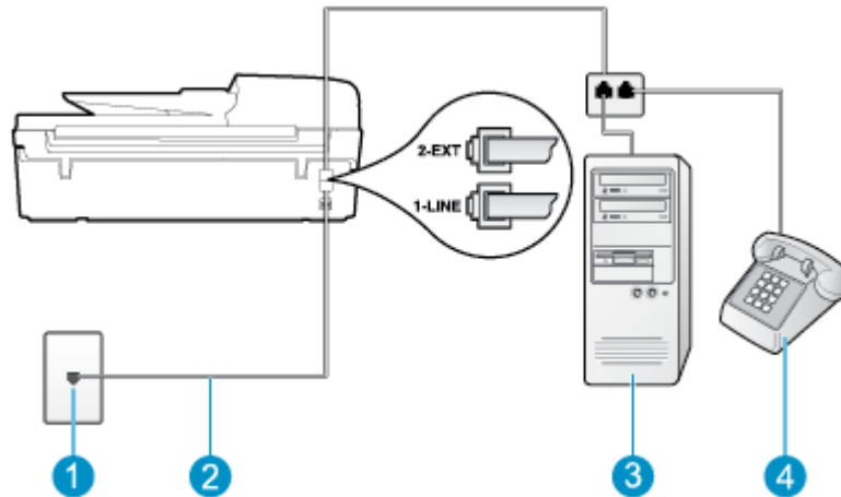
Gambar B-18 Tampak belakang printer
