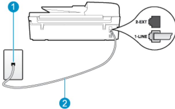
Gambar B-5 Tampak belakang printer
