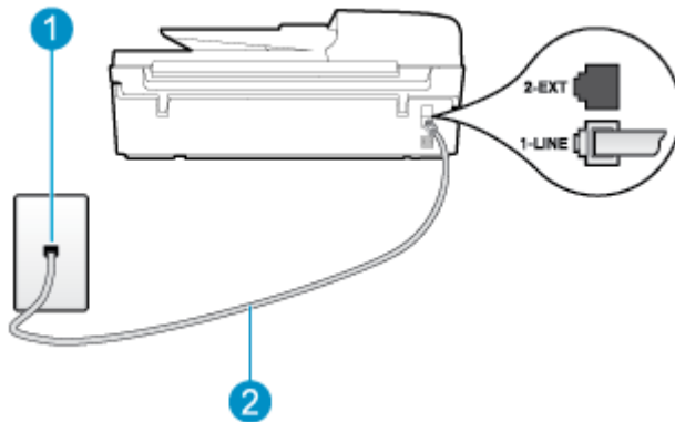
Gambar B-3 Tampak belakang printer
