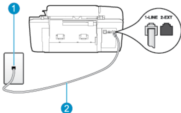
Фигура б-5 Изглед на принтера отзад
