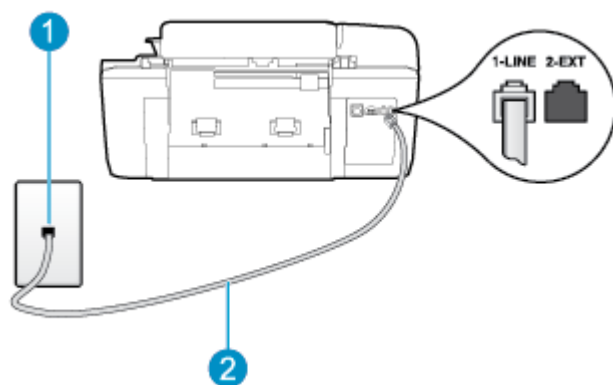
Фигура б-1 Изглед на принтера отзад
