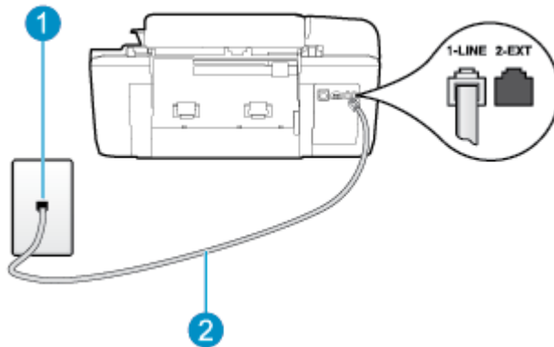
Gambar B-3 Tampilan belakang printer
