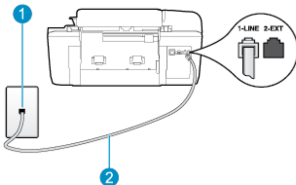
Gambar B-1 Tampilan belakang printer
