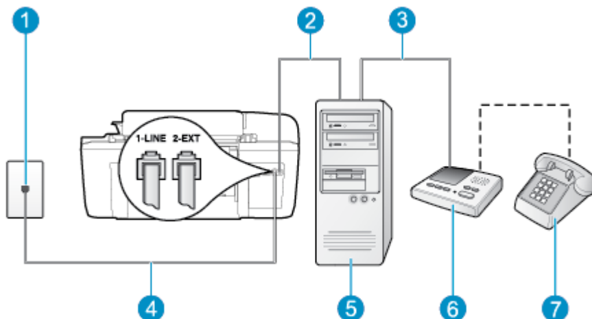
Сурет ә-14 Принтердің артқы көрінісі
