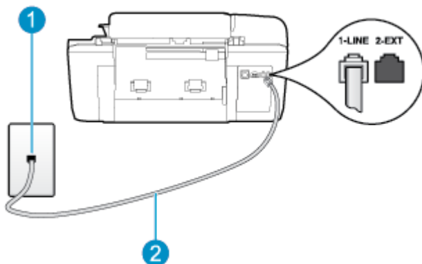
Сурет ә-5 Принтердің артқы көрінісі
