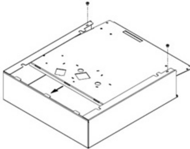
Abbildung 2-5 Entfernen des Gehäuses (hochbelastbare Kassenschublade)
