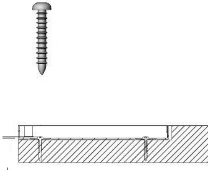
Abbildung 2-8 Sichern der Kassenschublade
