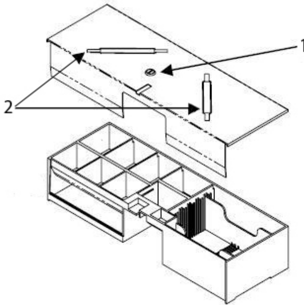
Abbildung 2-10 Entfernen der Einsatzabdeckung
