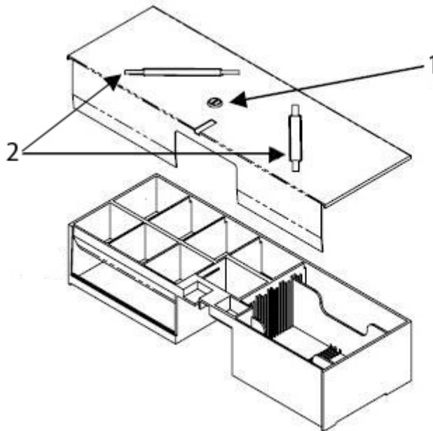
Figura 2-10 Extracción de la cubierta de la bandeja
