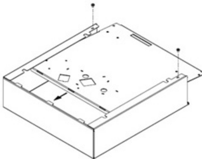
Figura 2-5 Extracción de la carcasa (caja de efectivo resistente)
