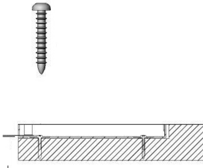
Figura 2-8 Fijación de la caja de efectivo
