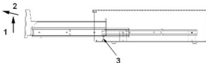
Figura 2-4 Extracción de la caja interna
