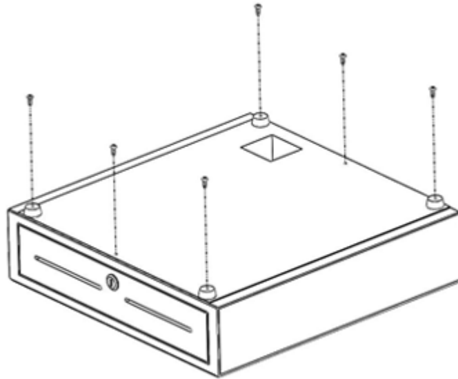
Figura 2-6 Extracción de la carcasa (caja de efectivo estándar)
