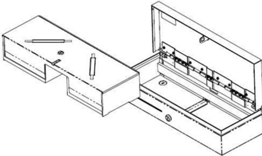
Figura 2-9 Extracción de la caja interna
