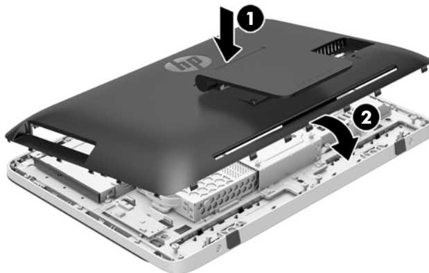
Figura 2-41 Reinstalação do painel de acesso
