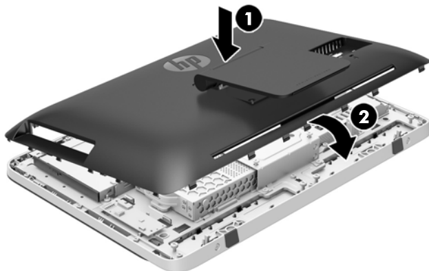
Figura 2-48 Reinstalação do painel de acesso
