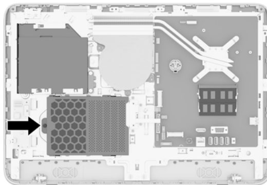
Figura 2-31 Localização do compartimento da unidade de disco rígido
