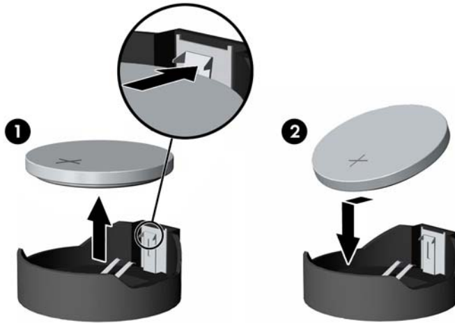
Figura 2-24 Remoção e substituição de uma bateria de lítio
