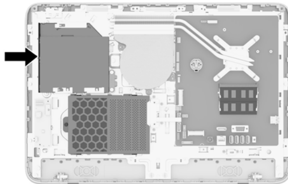
Figura 2-43 Localização da unidade de disco óptico
