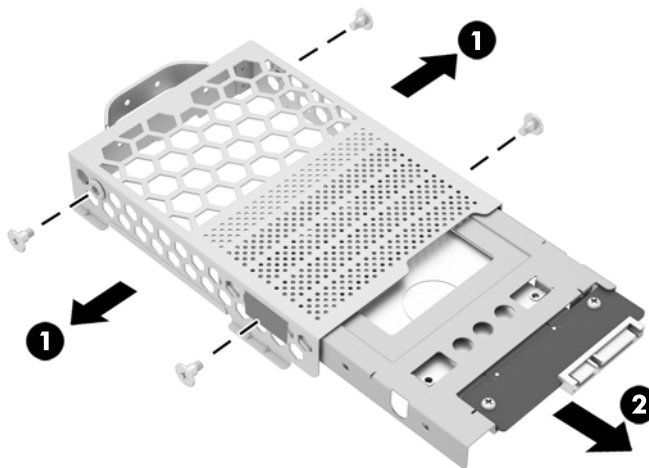
Figura 2-33 Remoção do compartimento da unidade
