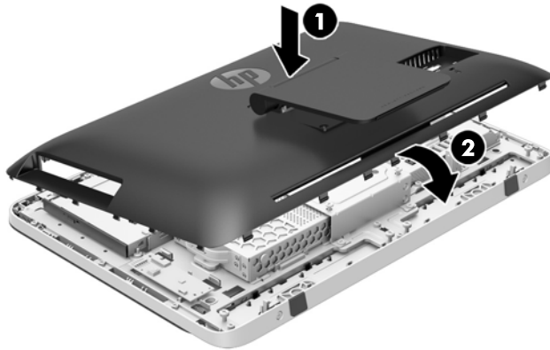
Figura 2-37 Reinstalação do painel de acesso
