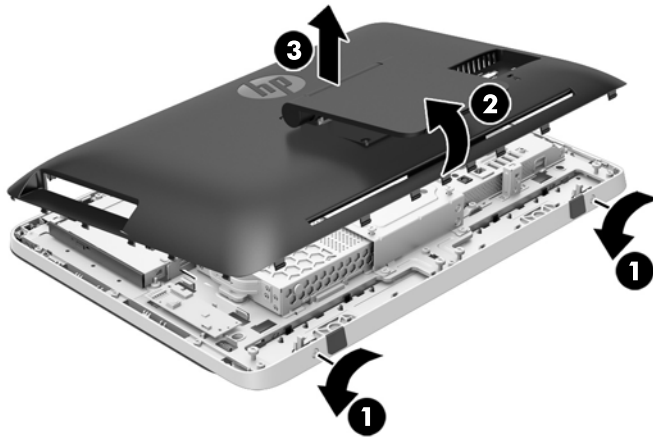
Figura 2-42 Remoção do painel de acesso
