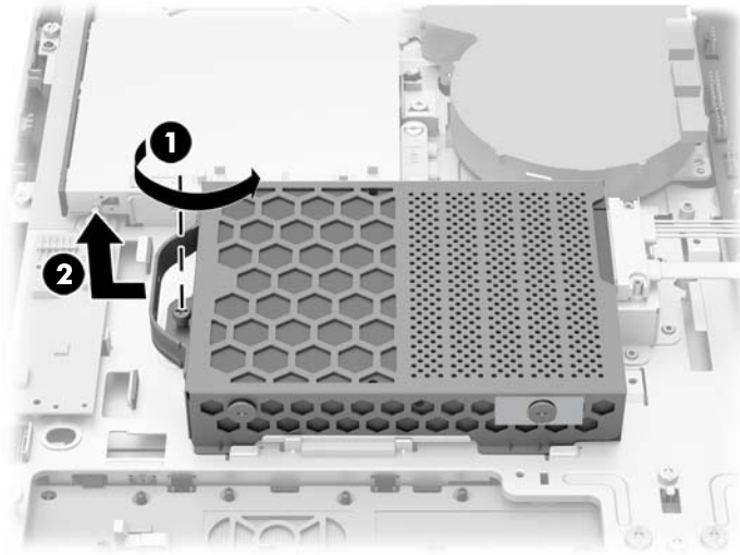
Figura 2-28 Remoção do compartimento da unidade de disco rígido
