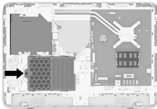
Figura 2-27 Localização do compartimento da unidade de disco rígido
