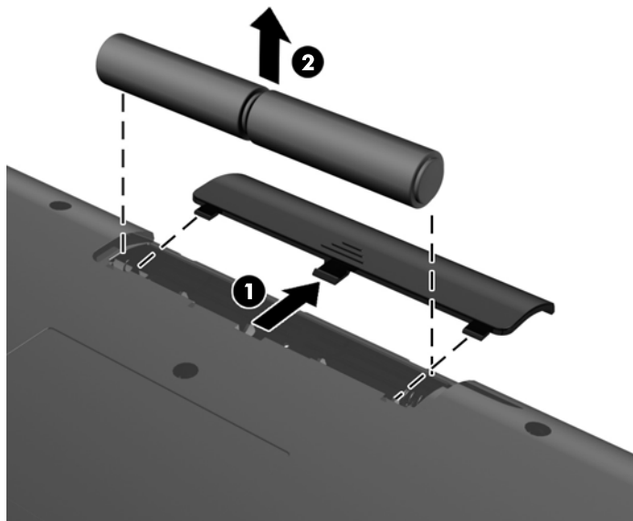
Figura 2-5 Remoção das baterias do teclado sem fio
