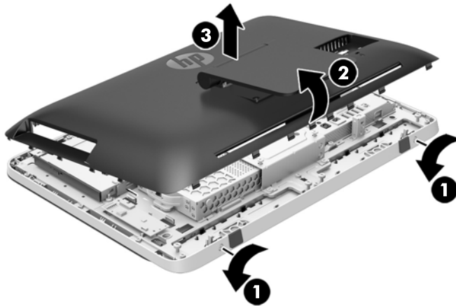
Figura 2-26 Remoção do painel de acesso
