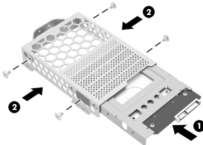
Figura 2-39 Instalação do adaptador de unidade de 2,5 polegadas no compartimento de unidade de disco rígido
