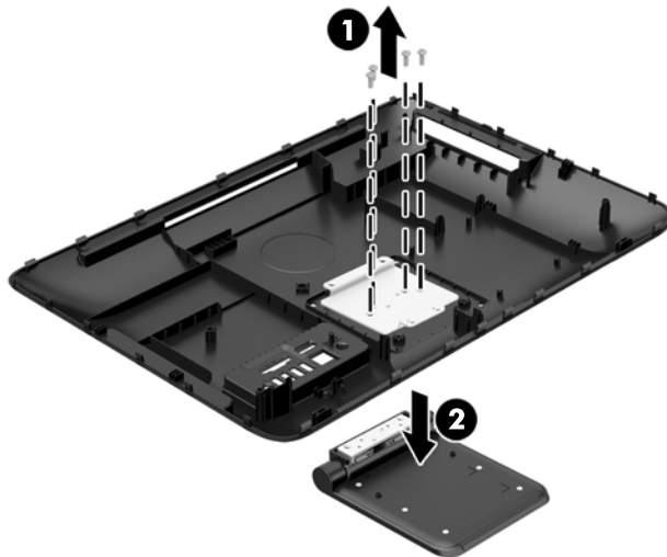
Figura 2-8 Remoção da base
