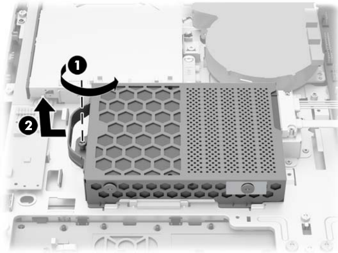
Figura 2-32 Remoção do compartimento da unidade de disco rígido
