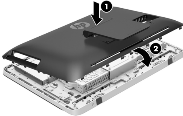
Figura 2-25 Reinstalação do painel de acesso
