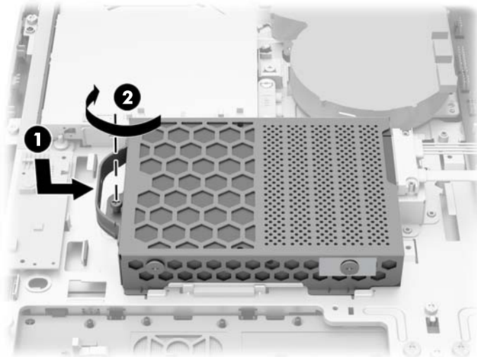
Figura 2-36 Instalação do compartimento da unidade de disco rígido
