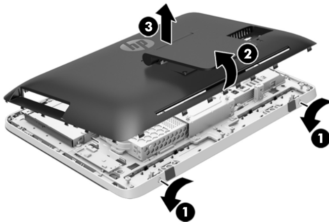
Figura 2-20 Remoção do painel de acesso
