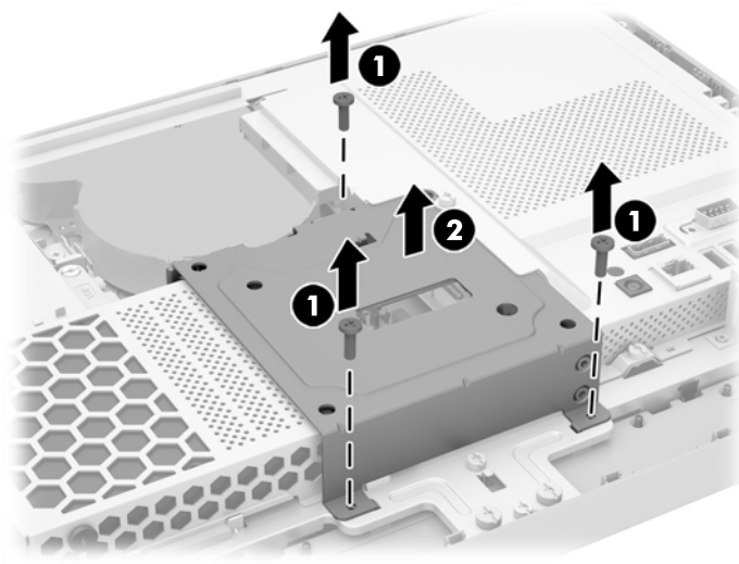
Figura 2-14 Remoção do painel VESA
