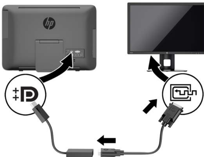
Figura 2-11 Conexão de um segundo monitor usando um adaptador DisplayPort
