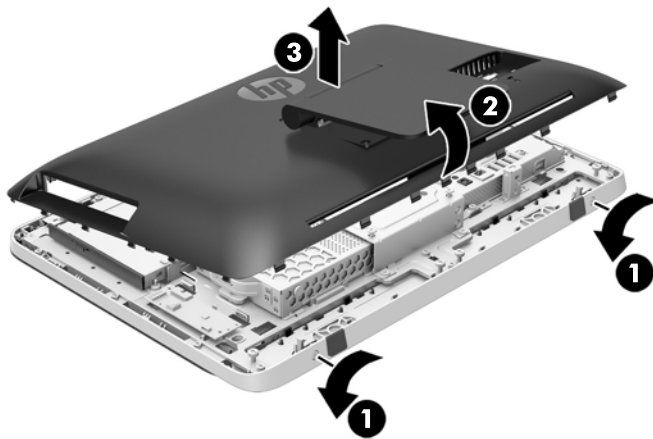
Figura 2-13 Remoção do painel de acesso
