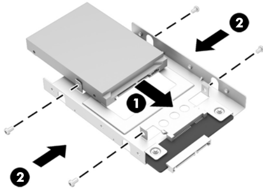
Figura 2-38 Montagem da unidade de disco rígido de 2,5 polegadas no adaptador
