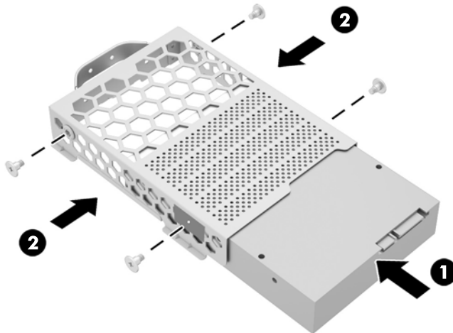
Figura 2-35 Instalação da unidade de disco rígido de 3,5 polegadas no compartimento de unidades de disco rígido
