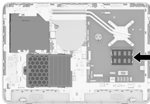
Figura 2-16 Localização dos módulos de memória
