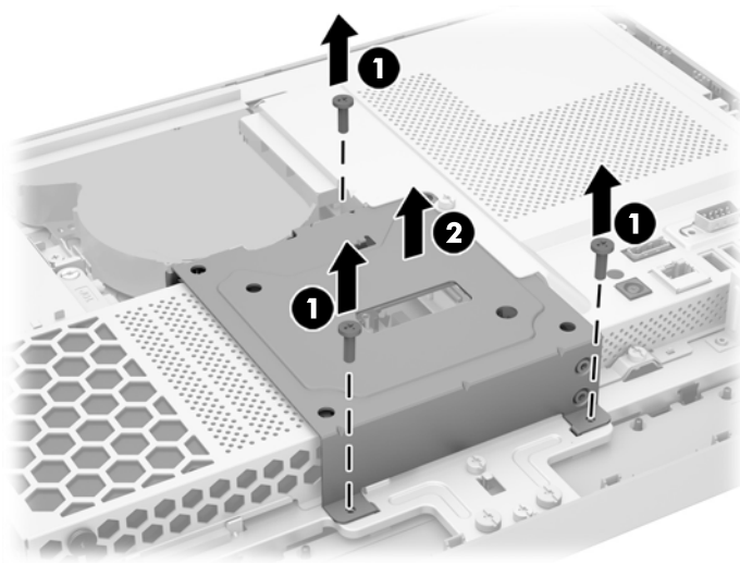
Figura 2-21 Remoção do painel VESA
