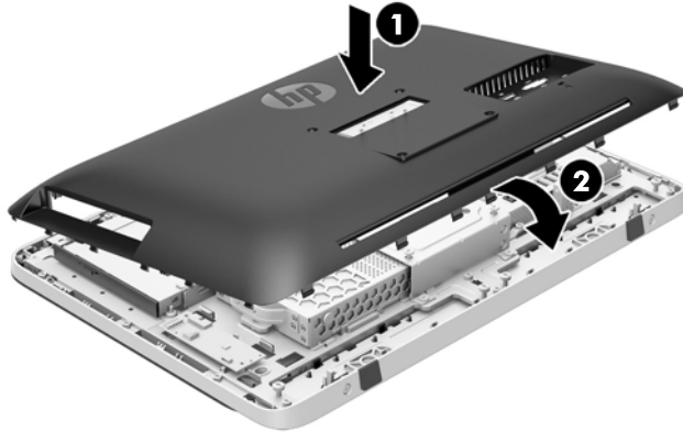
Figura 2-9 Reinstalação do painel de acesso
