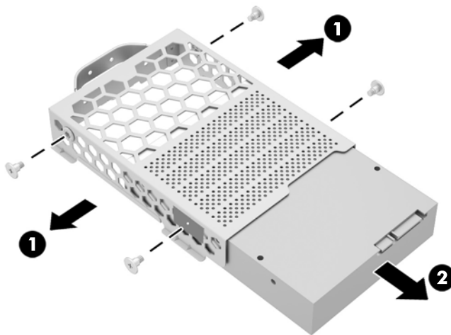
Figura 2-29 Remoção dos parafusos de montagem
