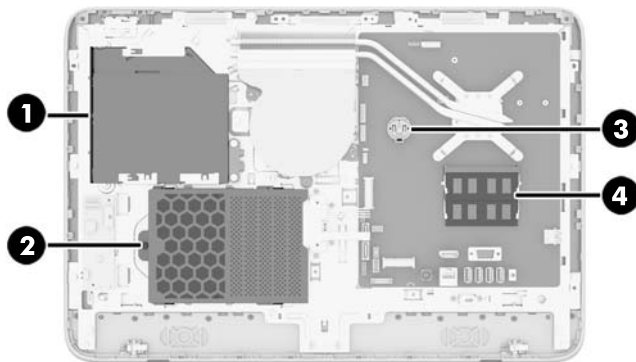
Figura 2-12 Localização dos componentes internos
