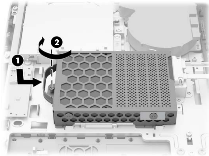
Figura 2-40 Instalação do compartimento da unidade de disco rígido
