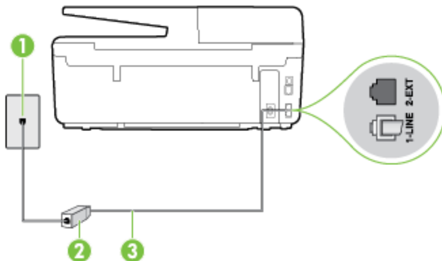
图 B-2 打印机的后视图
