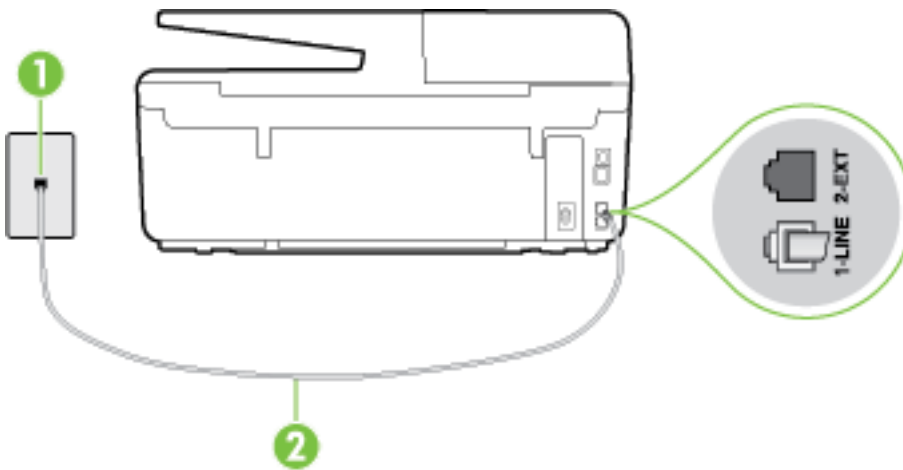
图 B-3 打印机的后视图
