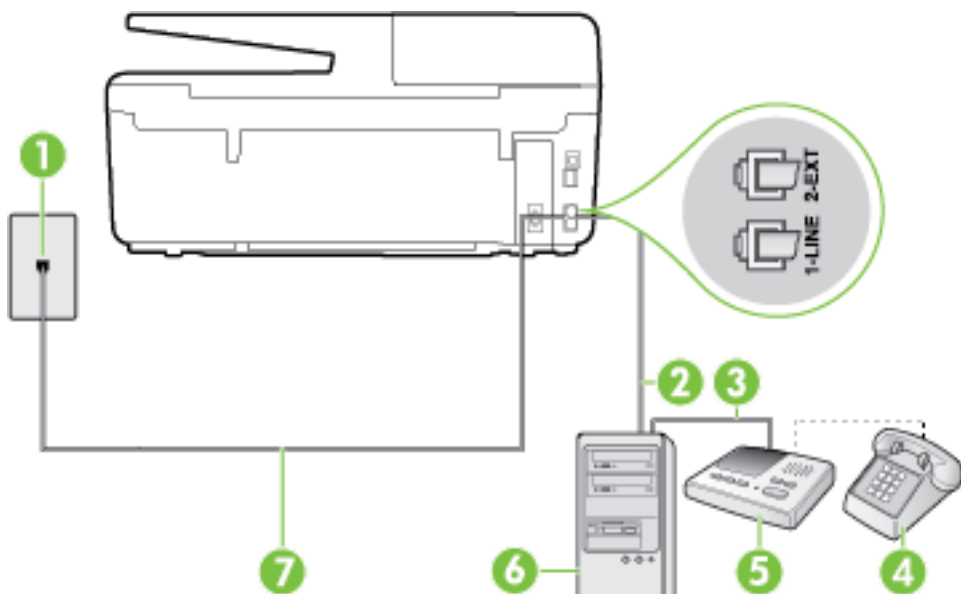
图 B-13 打印机的后视图
