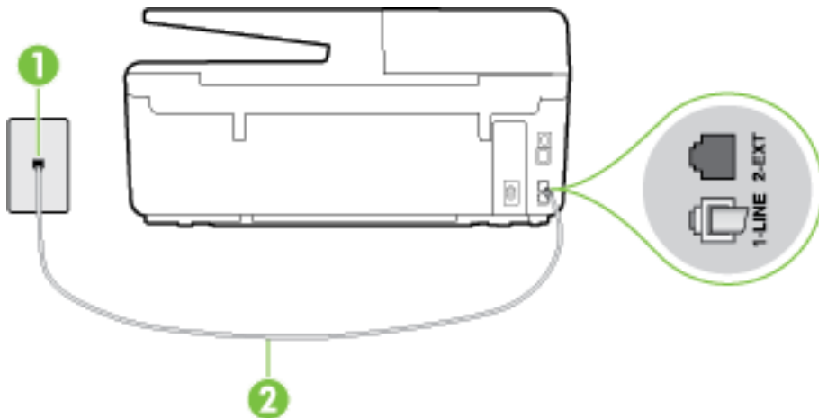
图 10-1 打印机的后视图
