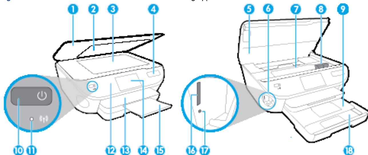
Figur 2-1 HP ENVY 5640 e-All-in-One series set forfra og oppefra
