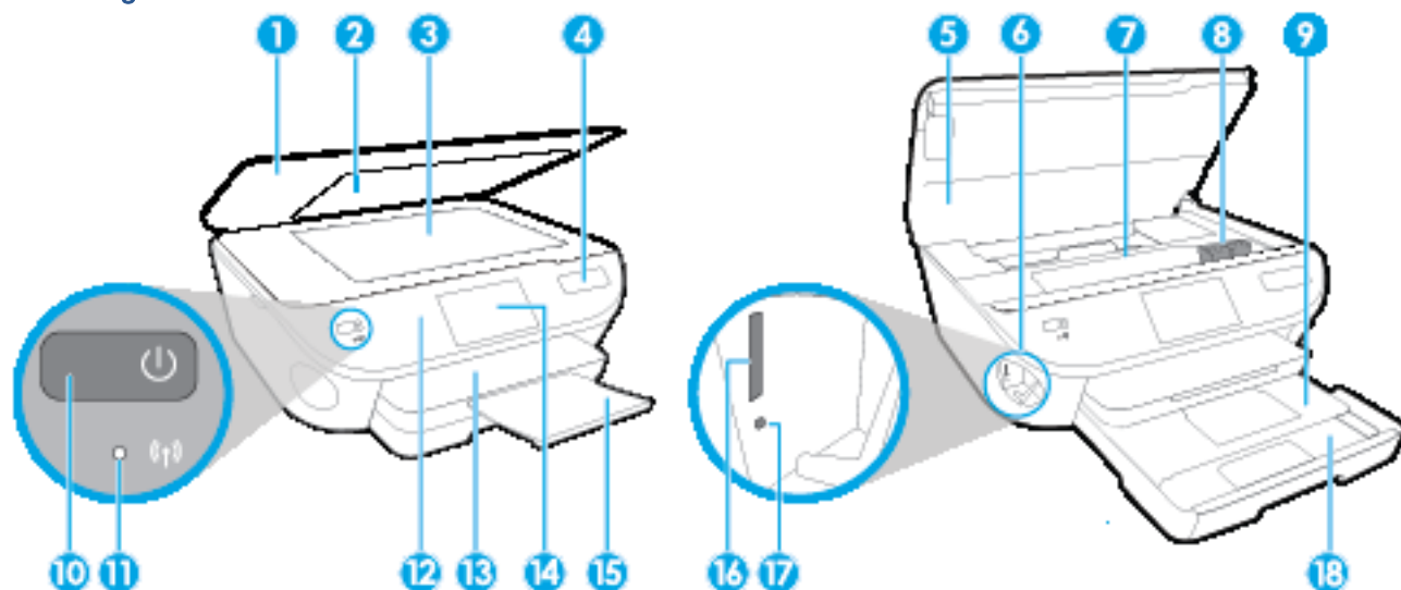
Afbeelding 2-1 Voor en bovenaanzicht van HP ENVY 5640 e-All-in-One series
