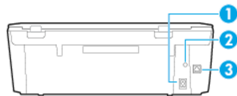
Figura 2-2 Vista posteriore di HP ENVY 5640 e-All-in-One series
