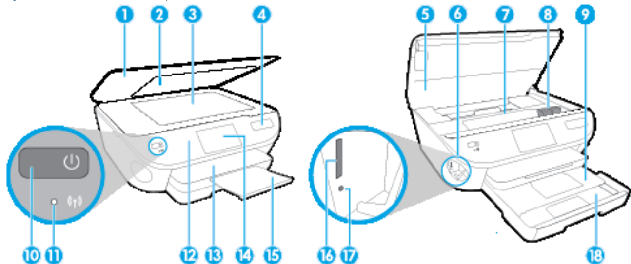
Figura 2-1 Viste anteriore e posteriore di HP ENVY 5640 e-All-in-One series
