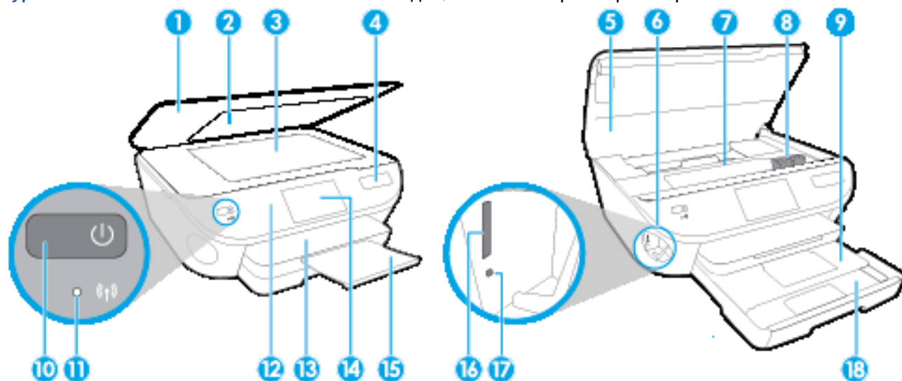
Сурет 2-1 HP ENVY 5640 e-All-in-One series алдыңғы және жоғарғы көріністері
