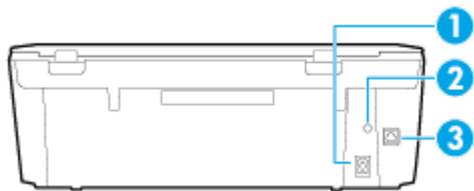
Сурет 2-2 HP ENVY 5640 e-All-in-One series артқы көрінісі
