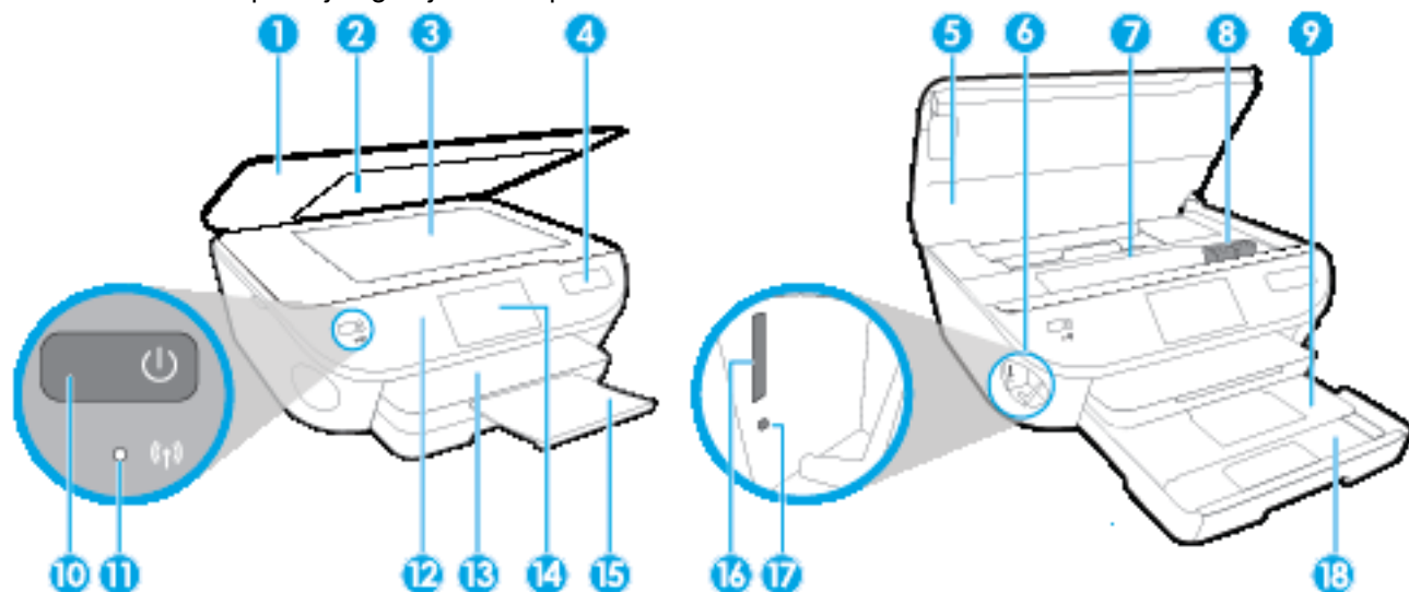
Slika 2-1 Prikazi s prednje i gornje strane proizvoda HP ENVY 5640 e-All-in-One series
