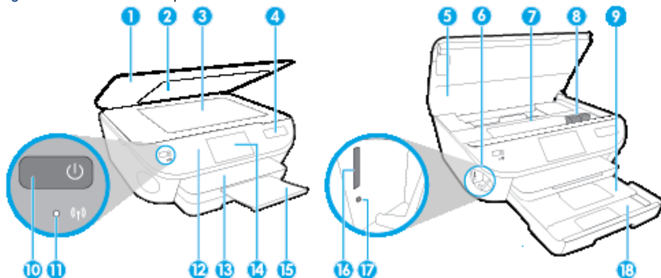
Figura 2-1 Viste anteriore e posteriore di HP ENVY 5660 e-All-in-One series
