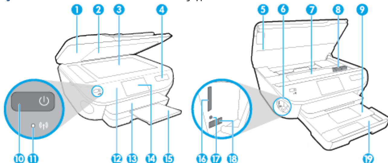
Figur 2-1 HP ENVY 7640 e-All-in-One-series set forfra og oppefra
