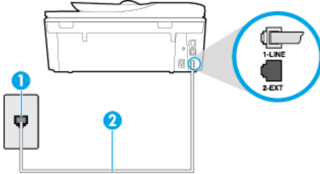
그림 9-1 프린터의 뒷 부분
