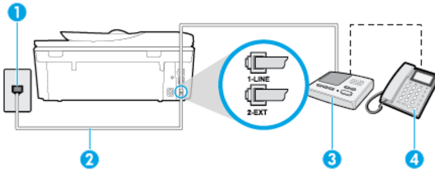
그림 B-11 프린터의 뒷 부분
