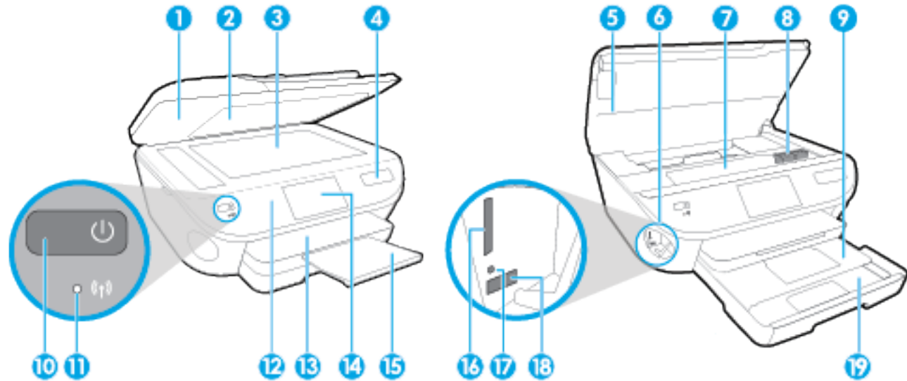
그림 2-1 HP ENVY 7640 e-All-in-One series의 앞면 및 윗면 뷰
