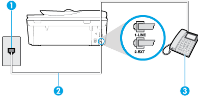
그림 B-4 프린터의 뒷 부분
