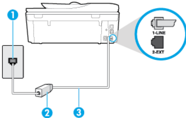
그림 B-2 프린터의 뒷 부분
