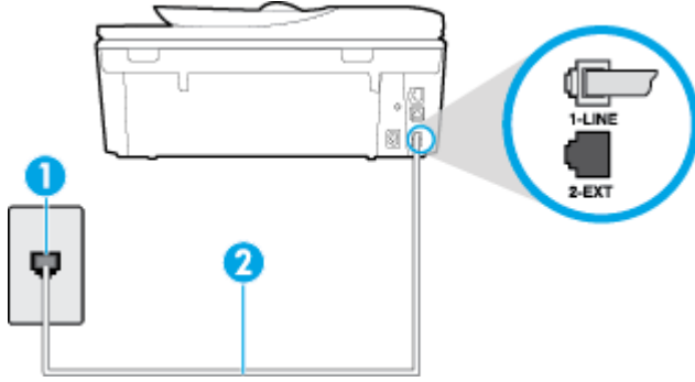
그림 B-3 프린터의 뒷 부분
