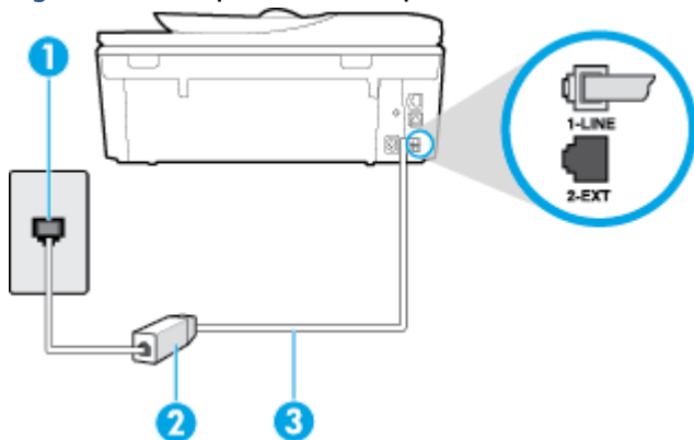
Figura B-2 Vista posterior do dispositivo
