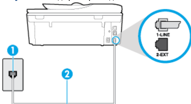
Рисунок Б-5 Вид принтера сзади
