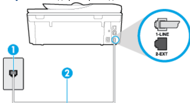
Рисунок Б-1 Вид принтера сзади
