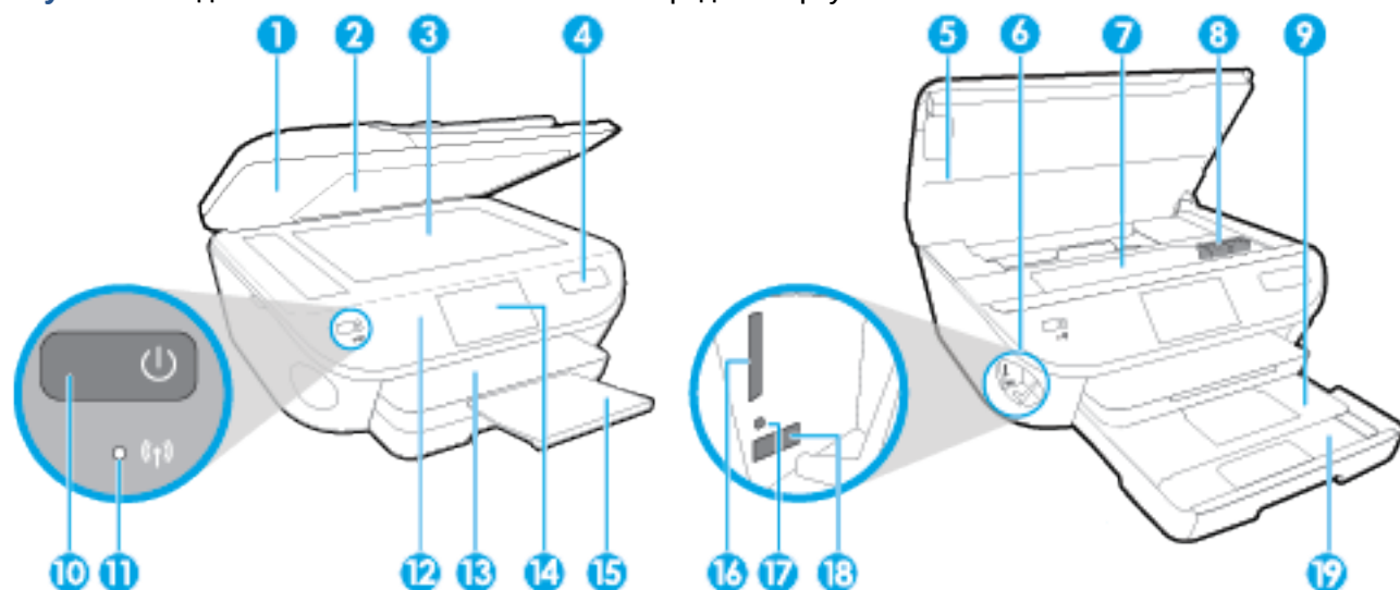
Рисунок 2-1 Вид HP ENVY 7640 e-All-in-One series спереди и сверху
