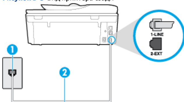
Рисунок Б-3 Вид принтера сзади
