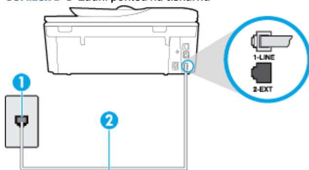
Obrázek B-5 Zadní pohled na tiskárnu
