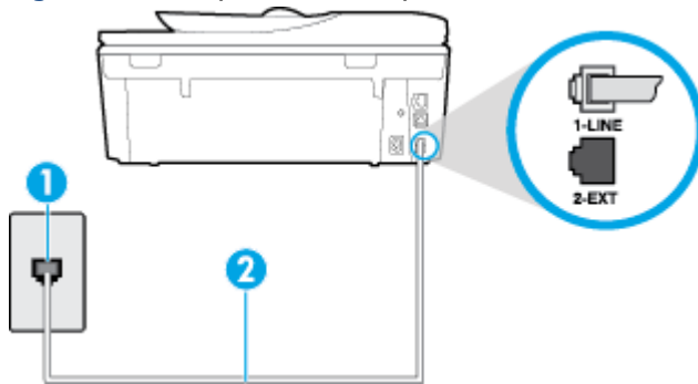
Figura 9-1 Vista posterior da impressora
