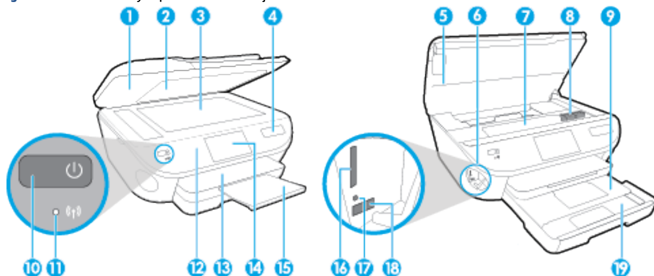
Figura 2-1 Vista frontal y superior de HP Officejet 5740 e-All-in-One series
