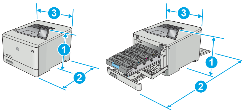
Figur 1-2 Mål for M452dn- og M452dw-modellerne
