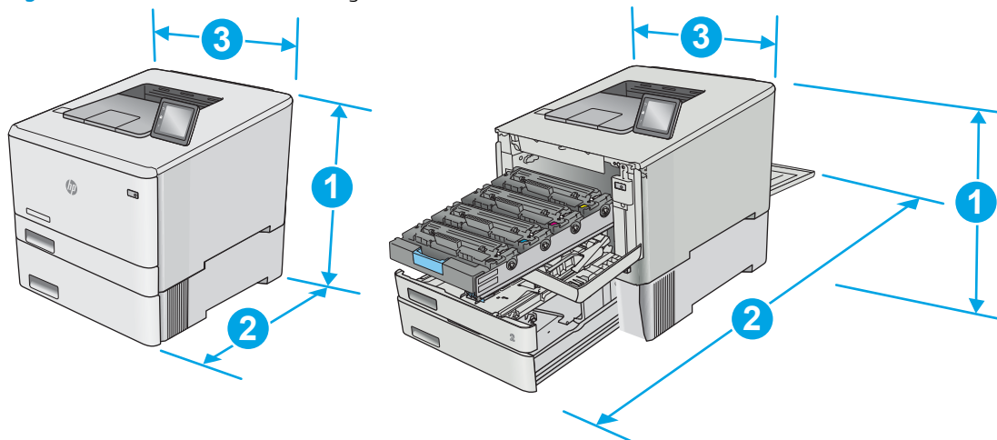
Figur 1-3 Mål for modeller med valgfri bakke 3
