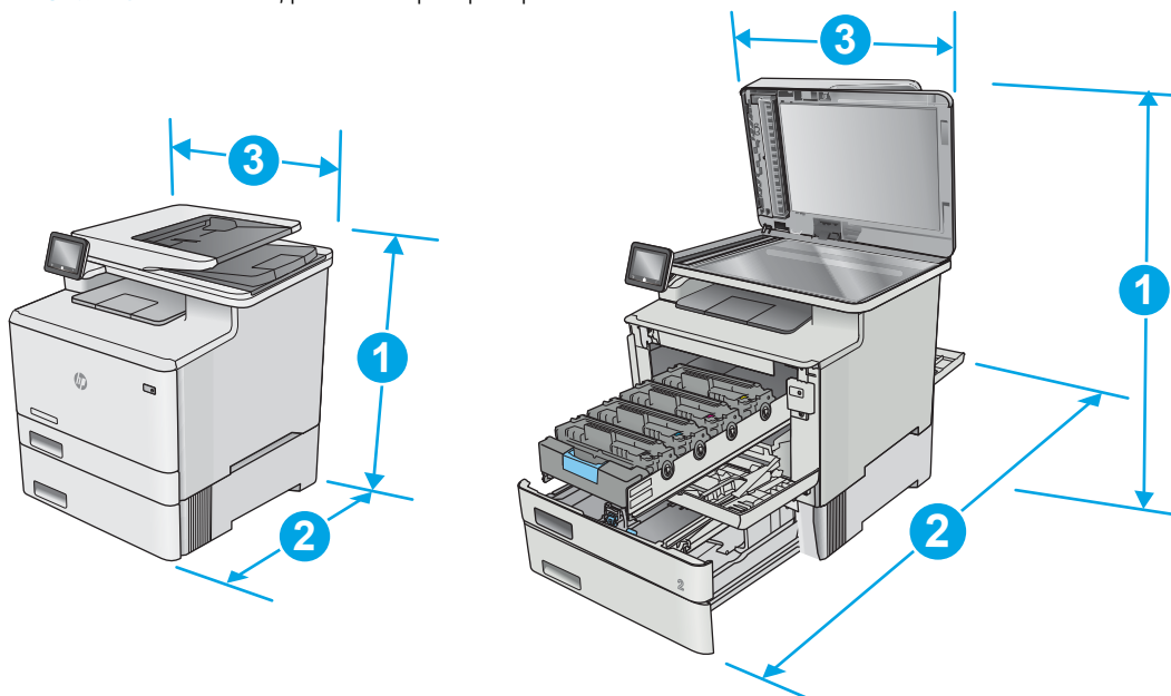
Εικόνα 1-3 Διαστάσεις μοντέλων με προαιρετικό Δίσκο 3
