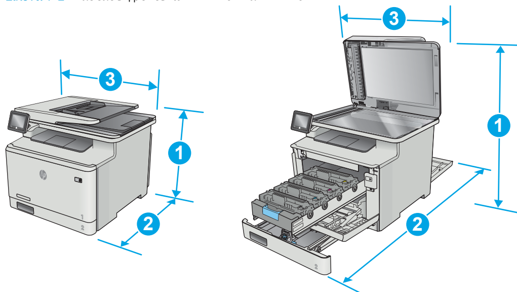
Εικόνα 1-2 Διαστάσεις μοντέλων M477fdn και M477fdw
