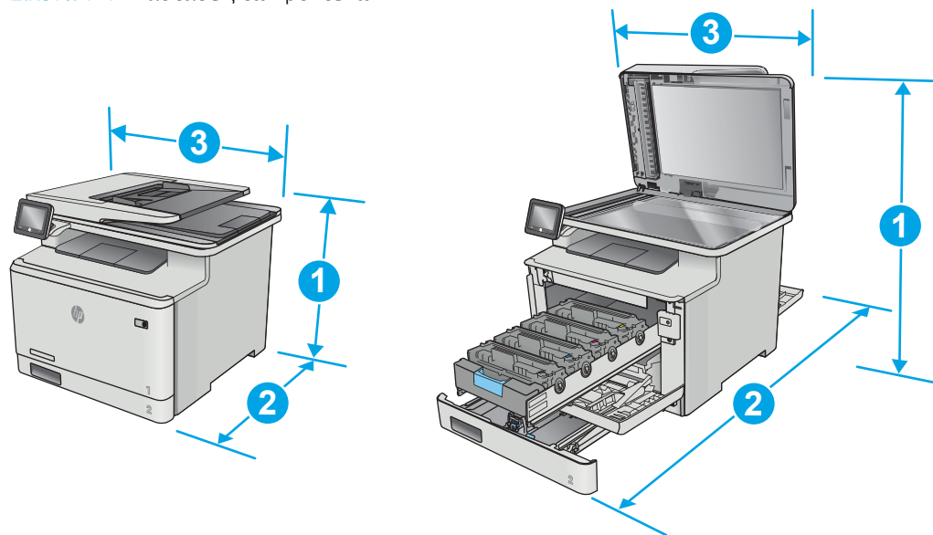
Εικόνα 1-1 Διαστάσεις των μοντέλων M477fnw
