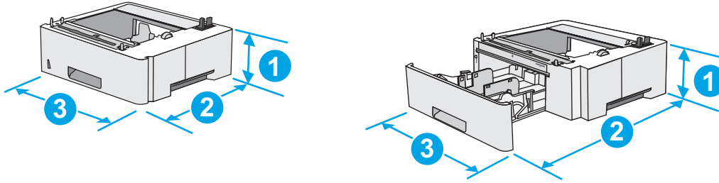
Figura 1-3 Dimensões para alimentador de papel 1 x 550 folhas
