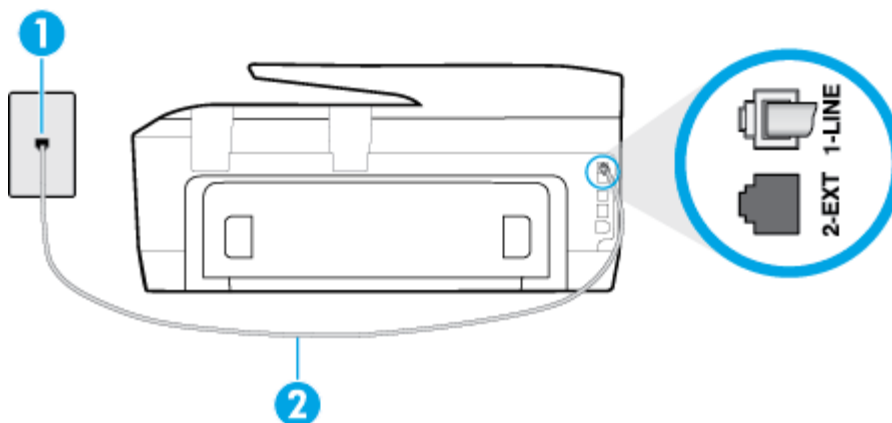
Фигура б-5 Изглед на принтера отзад
