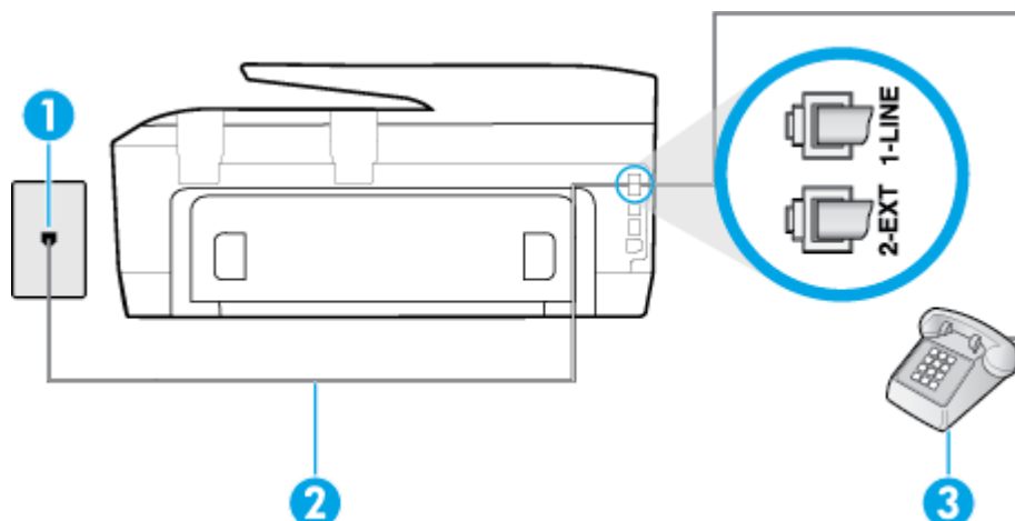
Фигура б-4 Изглед на принтера отзад
