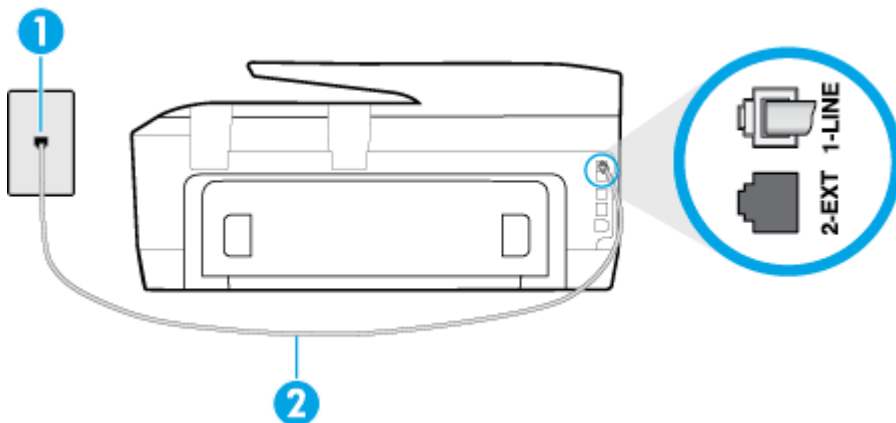
Фигура 10-1 Изглед на принтера отзад
