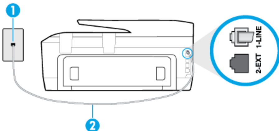
Obrázek 10-1 Zadní pohled na tiskárnu
