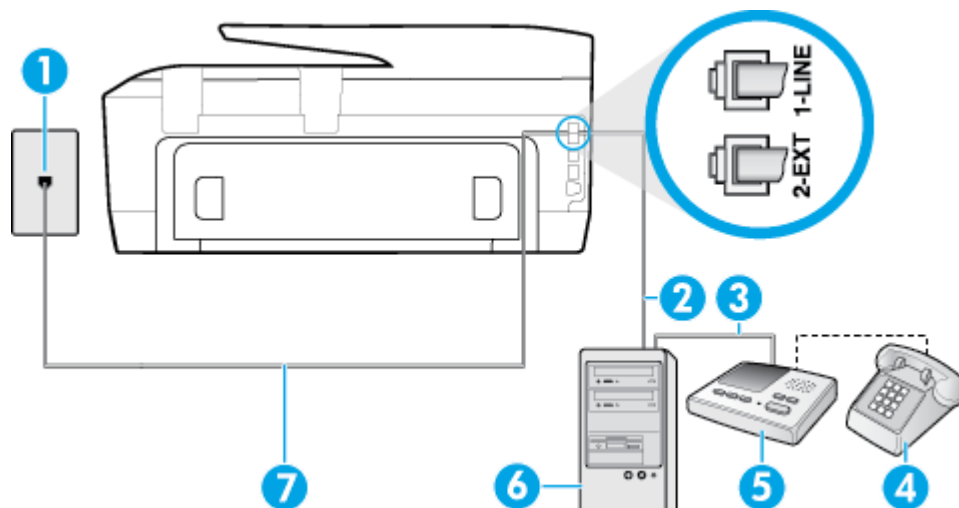
Obrázek B-13 Zadní pohled na tiskárnu
