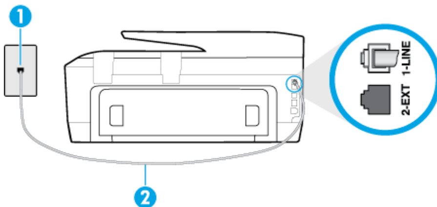
Obrázek B-3 Zadní pohled na tiskárnu
