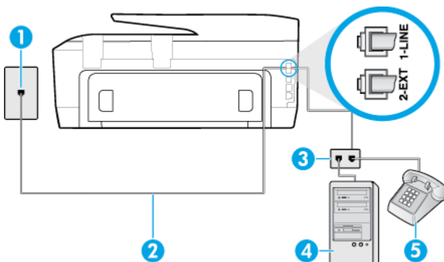
Obrázek B-9 Zadní pohled na tiskárnu
