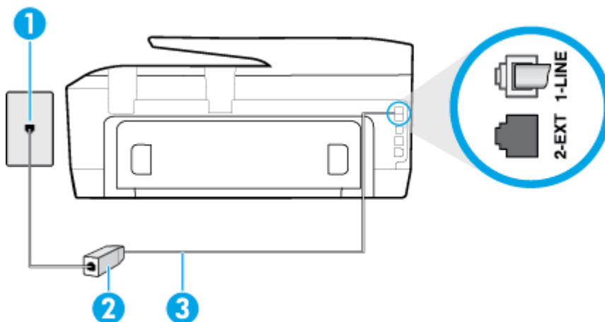
Obrázek B-2 Zadní pohled na tiskárnu
