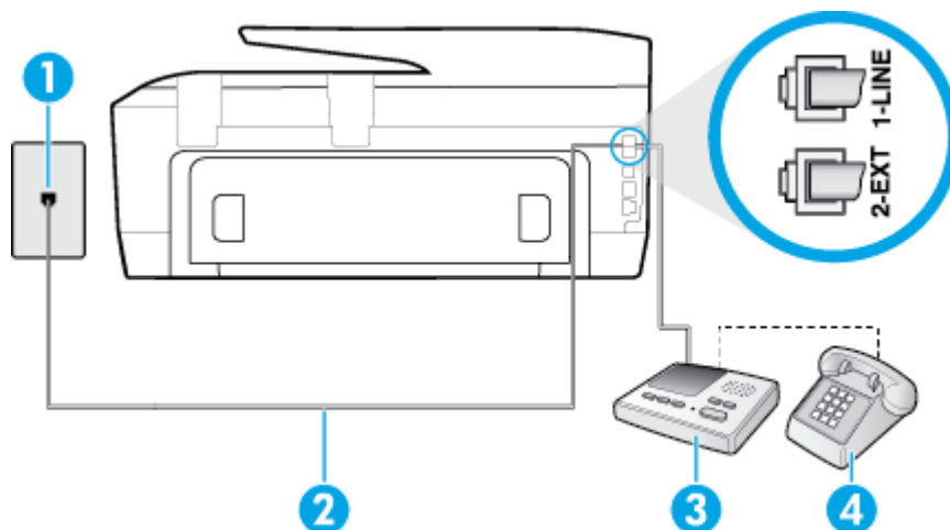
Obrázek B-11 Zadní pohled na tiskárnu
