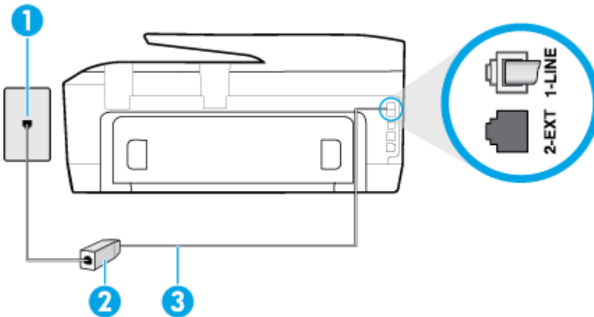
그림 B-2 프린터의 뒷 부분
