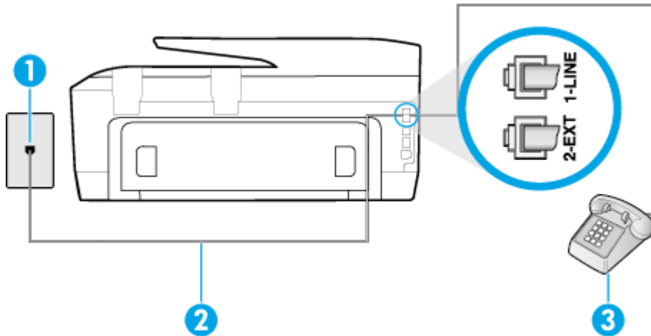
그림 B-4 프린터의 뒷 부분
