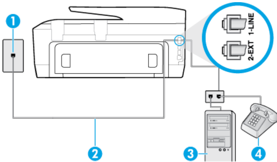
그림 B-16 프린터의 뒷 부분
