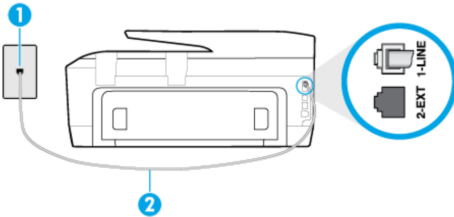
그림 B-5 프린터의 뒷 부분
