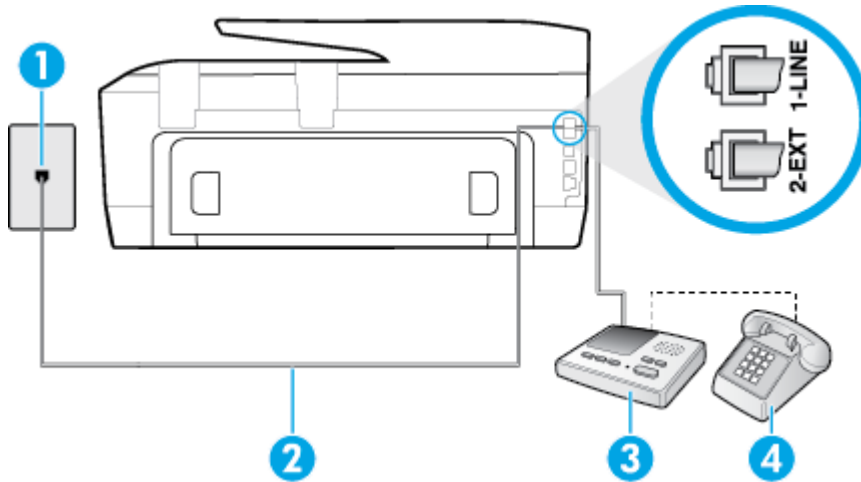
그림 B-11 프린터의 뒷 부분
