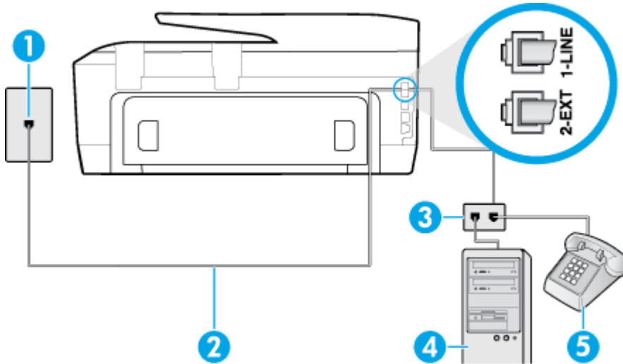
그림 B-9 프린터의 뒷 부분
