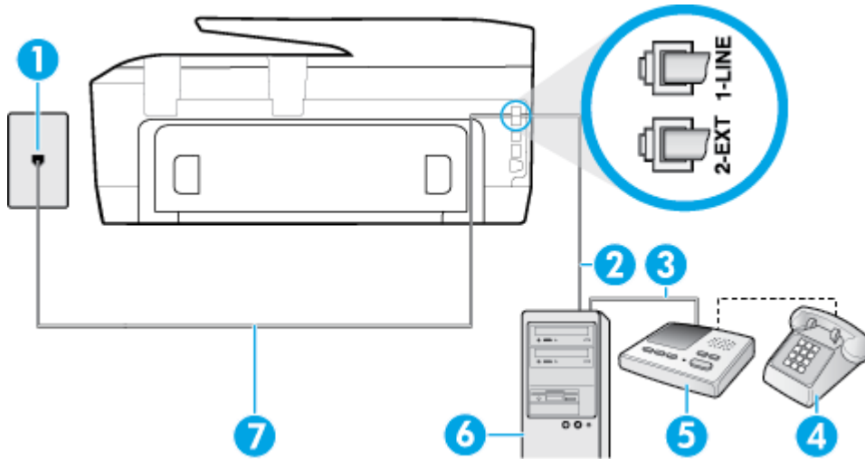
그림 B-13 프린터의 뒷 부분
