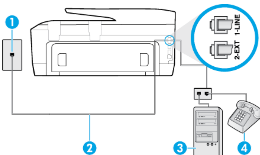
圖示 B-16 印表機的背視圖
