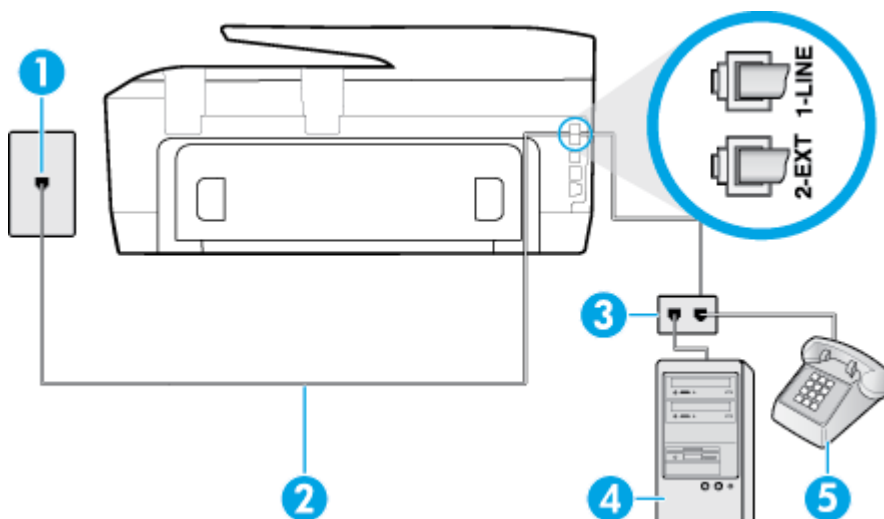
圖示 B-9 印表機的背視圖
