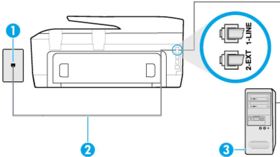
圖示 B-6 印表機的背視圖
