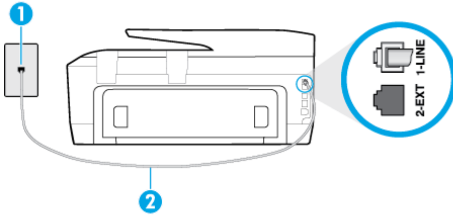
圖示 10-1 印表機的背視圖
