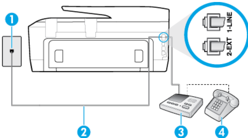
圖示 B-11 印表機的背視圖
