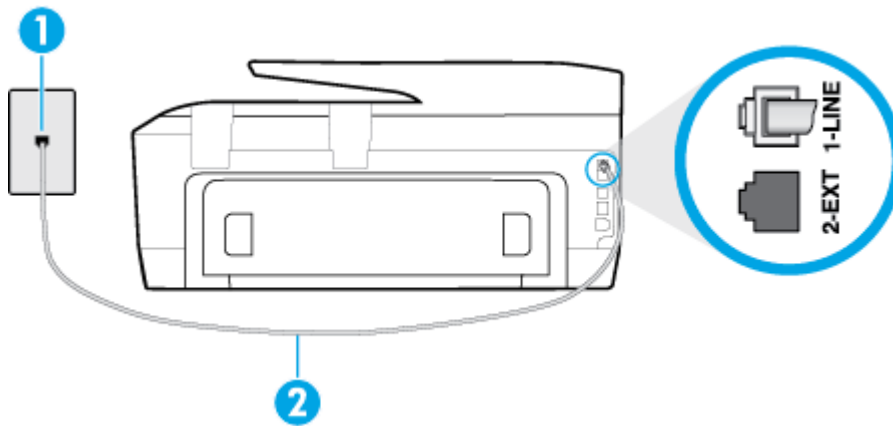
圖示 B-3 印表機的背視圖
