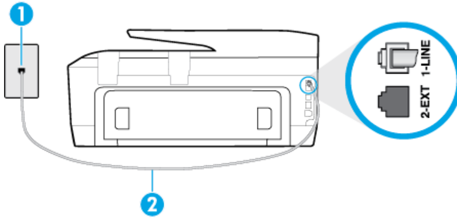
圖示 B-1 印表機的背視圖
