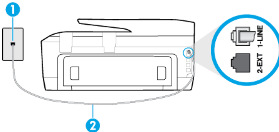
Рисунок 6-5 Задня панель принтера
