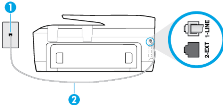
Рисунок 10-1 Задня панель принтера
