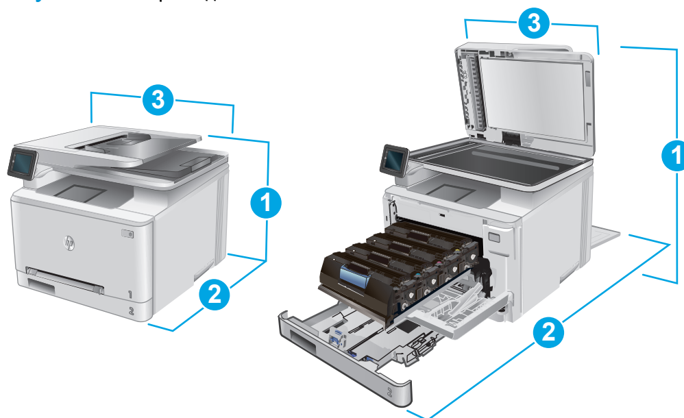
Рисунок 1-1 Размеры модели M274n
