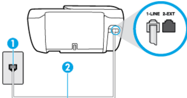
Gambar B-1 Tampilan belakang printer
