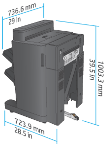
Tabuľka 1-19 Priestorové požiadavky pre zariadenie a pripojené dokončovacie príslušenstvo, keď sú všetky dvierka, zásobníky a podávač dokumentov úplne otvorené
