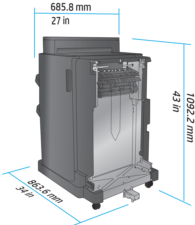
Tabuľka 1-9 Priestorové požiadavky pre zariadenie a pripojené príslušenstvo, keď sú všetky dverka, zásobníky a podávač dokumentov úplne otvorené
