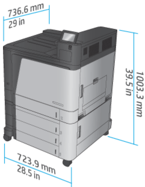
Tabuľka 1-12 Priestorové požiadavky, keď sú všetky dverka a zásobníky úplne otvorené
