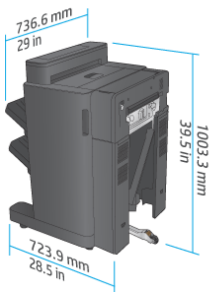
Tabuľka 1-14 Priestorové požiadavky pre zariadenie a pripojené dokončovacie príslušenstvo, keď sú všetky dvierka a zásobníky úplne otvorené
