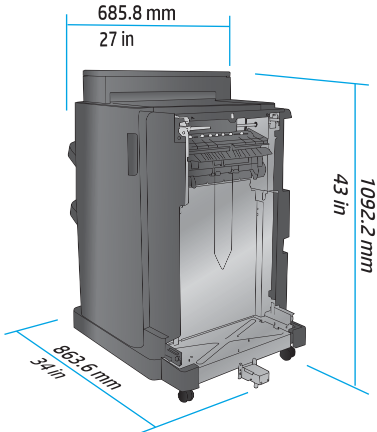
Tabuľka 1-4 Priestorové požiadavky pre zariadenie a pripojené príslušenstvo, keď sú všetky dvierka a zásobníky úplne otvorené
