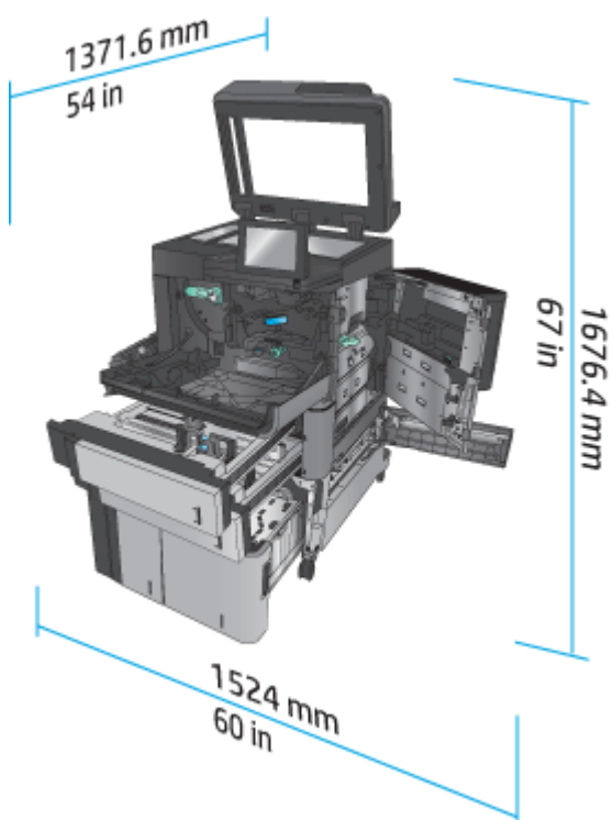
Obrázok 1-8 Priestorové požiadavky, keď sú všetky dverka, zásobníky a podávač dokumentov úplne otvorené
