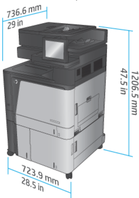
Obrázok 1-17 Rozmery zariadenia, keď sú všetky dverka, zásobníky a podávač dokumentov zatvorené
