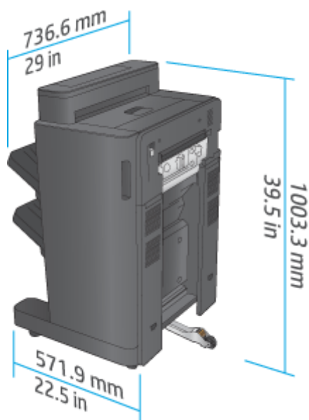
Obrázok 1-13 Rozmery dokončovacieho príslušenstva, keď sú všetky dvierka a zásobníky zatvorené
