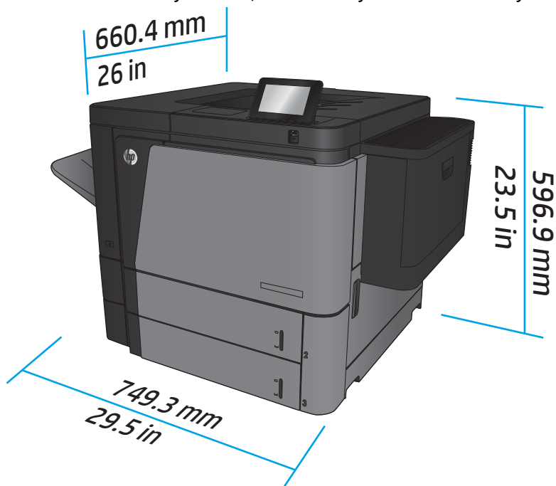
Obrázok 1-1 Rozmery M806dn, keď sú všetky dvierka a zásobníky zatvorené
