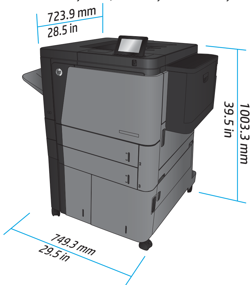
Tabuľka 1-2 Priestorové požiadavky, keď sú všetky dvierka a zásobníky úplne otvorené
