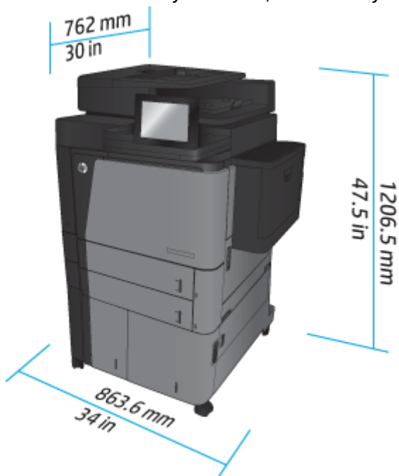
Tabuľka 1-7 Priestorové požiadavky, keď sú všetky dverka, zásobníky a podávač dokumentov úplne otvorené
