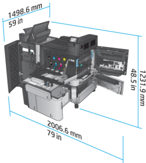
Obrázok 1-15 Priestorové požiadavky pre zariadenie a pripojené dokončovacie príslušenstvo, keď sú všetky dvierka a zásobníky úplne otvorené
