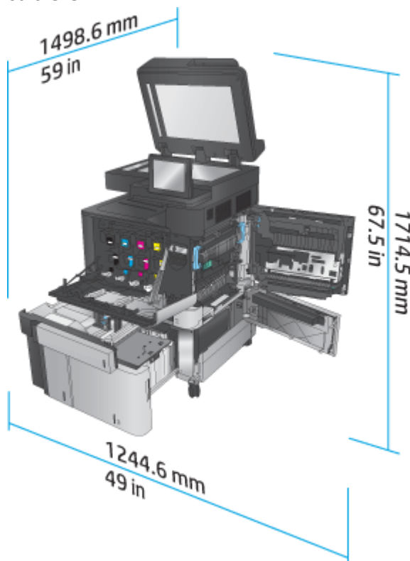
Tabuľka 1-18 Rozmery príslušenstva, keď sú všetky dvierka zatvorené
