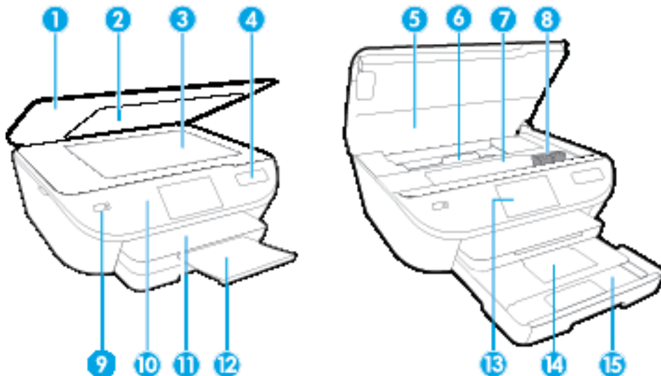
図 2-1 HP ENVY 5540 All-in-One series の正面および上面図
