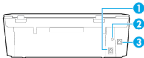
図 2-2 HP ENVY 5540 All-in-One series の背面図
