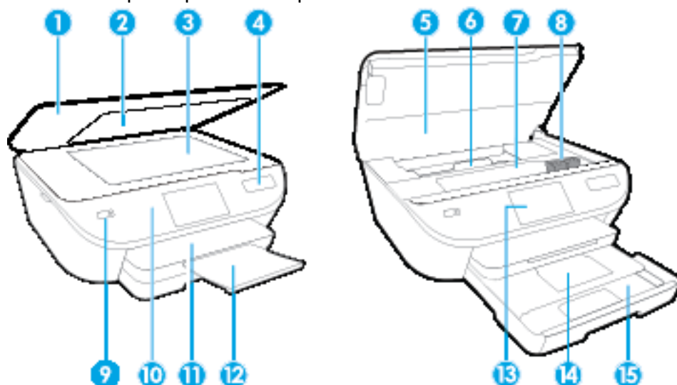
Εικόνα 2-1 Μπροστινή και άνω πλευρά του HP DeskJet 5570 All-in-One series
