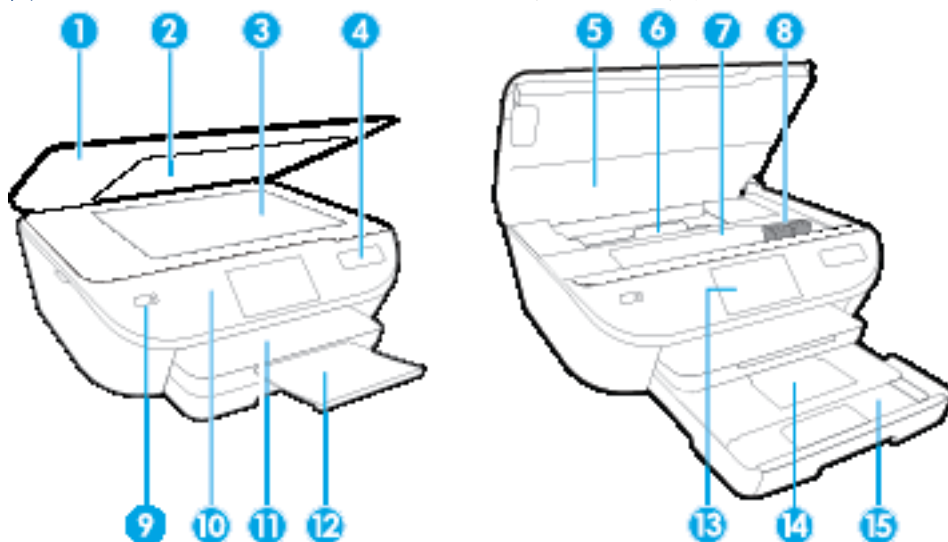
図 2-1 HP DeskJet 5570 All-in-One series の正面および上面図
