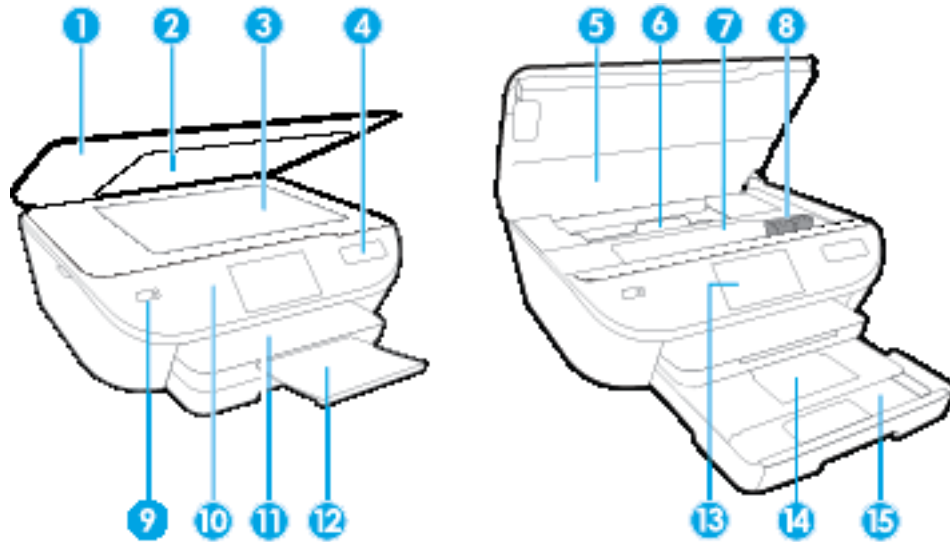
그림 2-1 HP DeskJet 5570 All-in-One series 의 앞면 및 윗면 뷰
