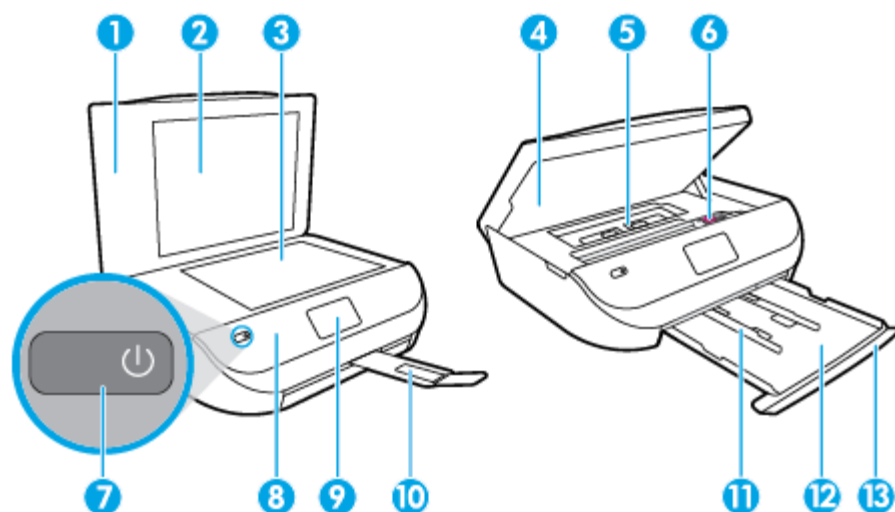
Afbeelding 2-1 Voor en bovenaanzicht van HP DeskJet Ink Advantage 4530 All-in-One series
