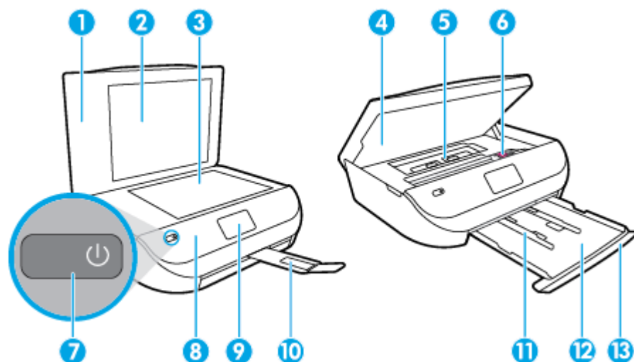
図 2-1 HP DeskJet Ink Advantage 4530 All-in-One series の正面および上面図
