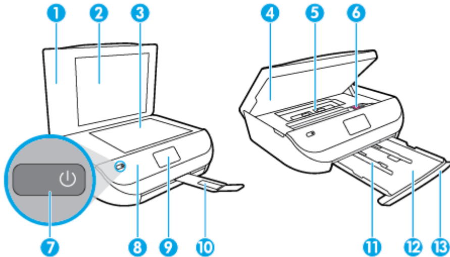
ภาพ 2-1 มุมมองด้านหน้าและด้านบนของ HP DeskJet Ink Advantage 4530 All-in-One series
