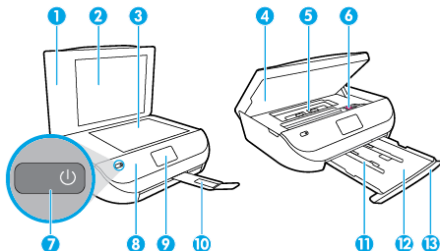
圖示 2-1 HP DeskJet Ink Advantage 4530 All-in-One series 的前視圖與俯視圖
