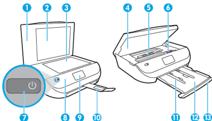
圖示 2-1 HP ENVY 4510 All-in-One series 的前視圖與俯視圖
