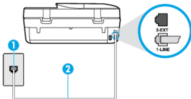
Slika B-3 Prikaz stražnje strane pisaa
