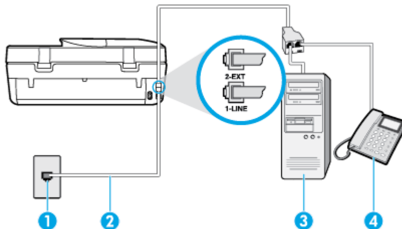
Abbildung B-16 Rückansicht des Druckers
