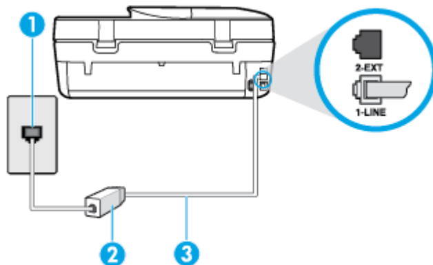
Abbildung B-2 Rückansicht des Druckers
