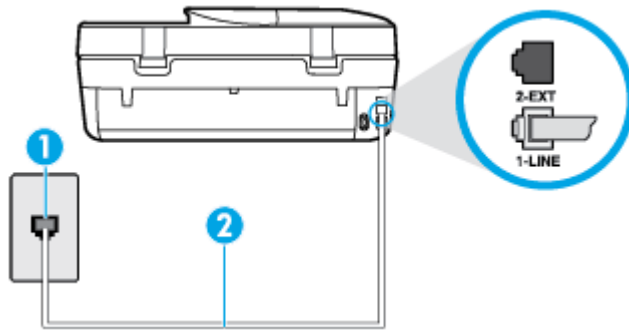
그림 B-5 프린터의 뒷 부분
