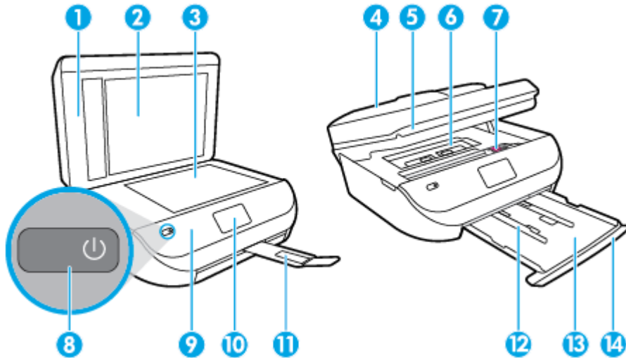
그림 2-1 HP OfficeJet 4650 All-in-One series의 앞면 및 윗면 뷰
