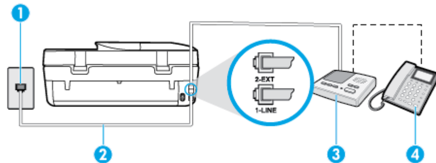
그림 B-11 프린터의 뒷 부분
