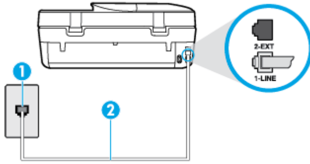
그림 B-1 프린터의 뒷 부분
