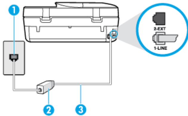
그림 B-2 프린터의 뒷 부분
